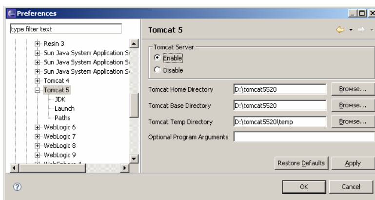
图 3.9 整合 Tomcat5
