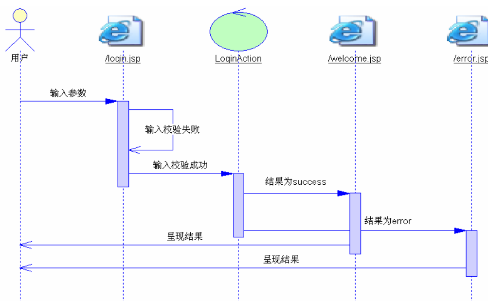
图 3.2 系统顺序图
