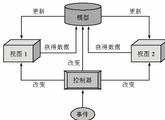
图 1.6 MVC 结构
