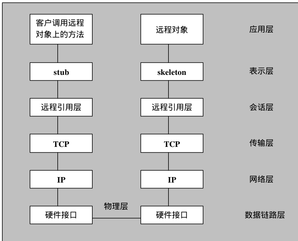
图 5 RMI 分层
