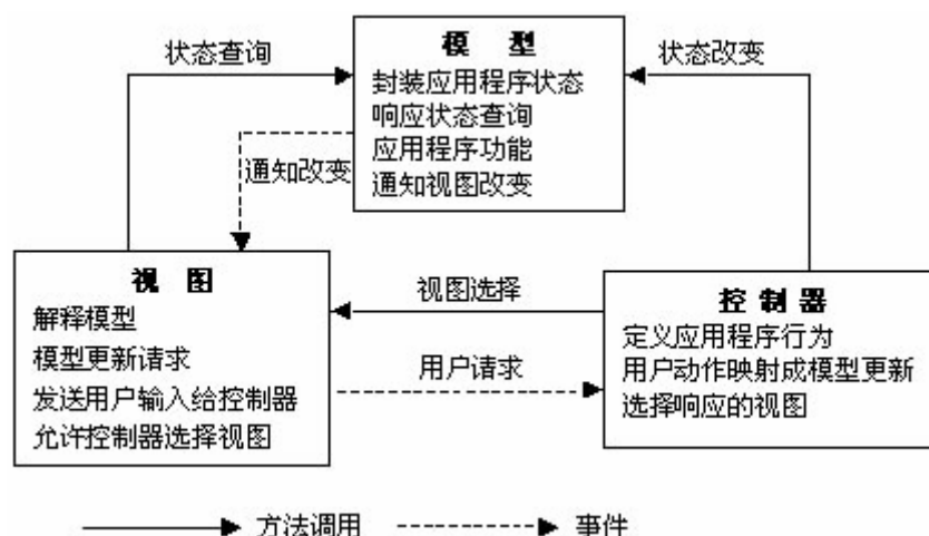
图 9.1 MVC 结构图
