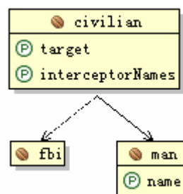
图 10.9 Bean 关系图
