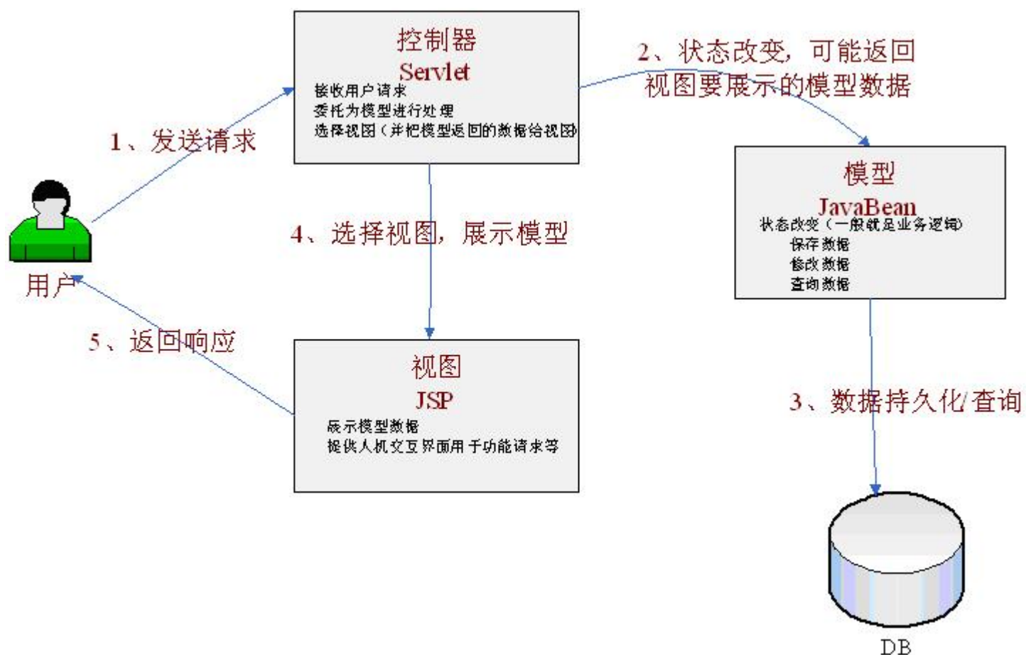
图1-9 Model2架构
