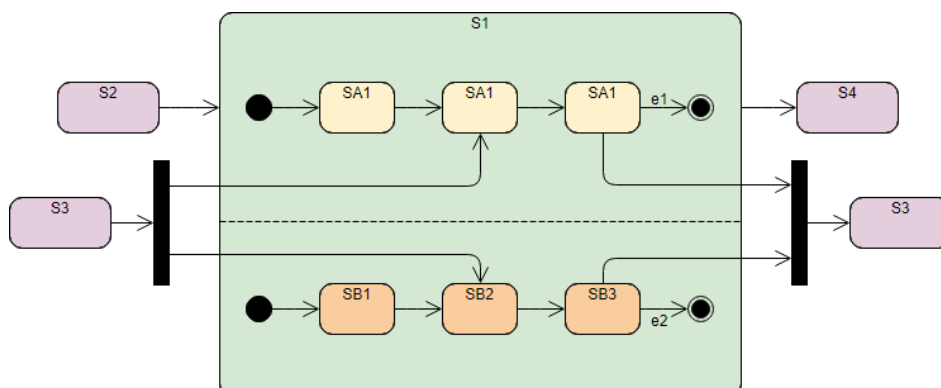
图 9：正交状态（图片来自 visual paradigm）
