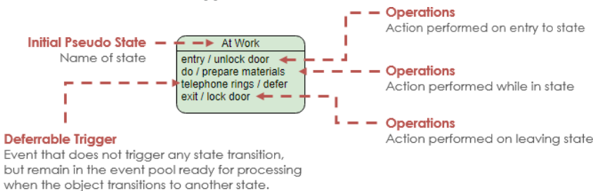
图 1：状态（图片来自 visual paradigm）
