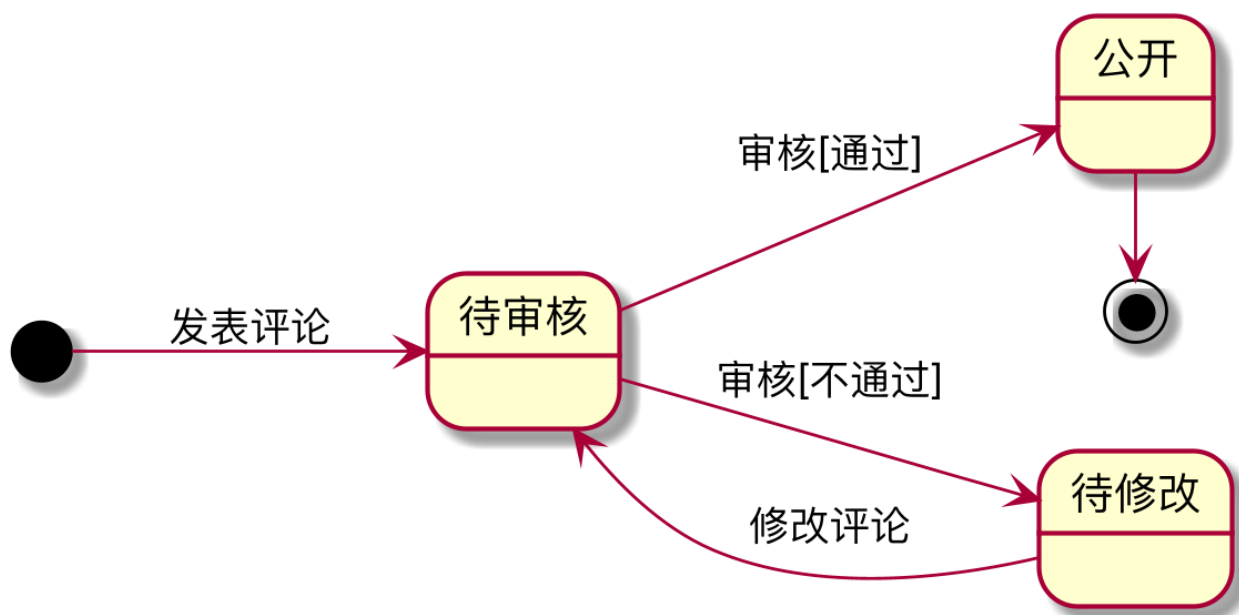
图 12: 评论审核状态图
