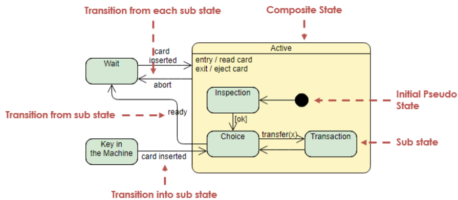
图 7：状态机图终止（图片来自 visual paradigm）
