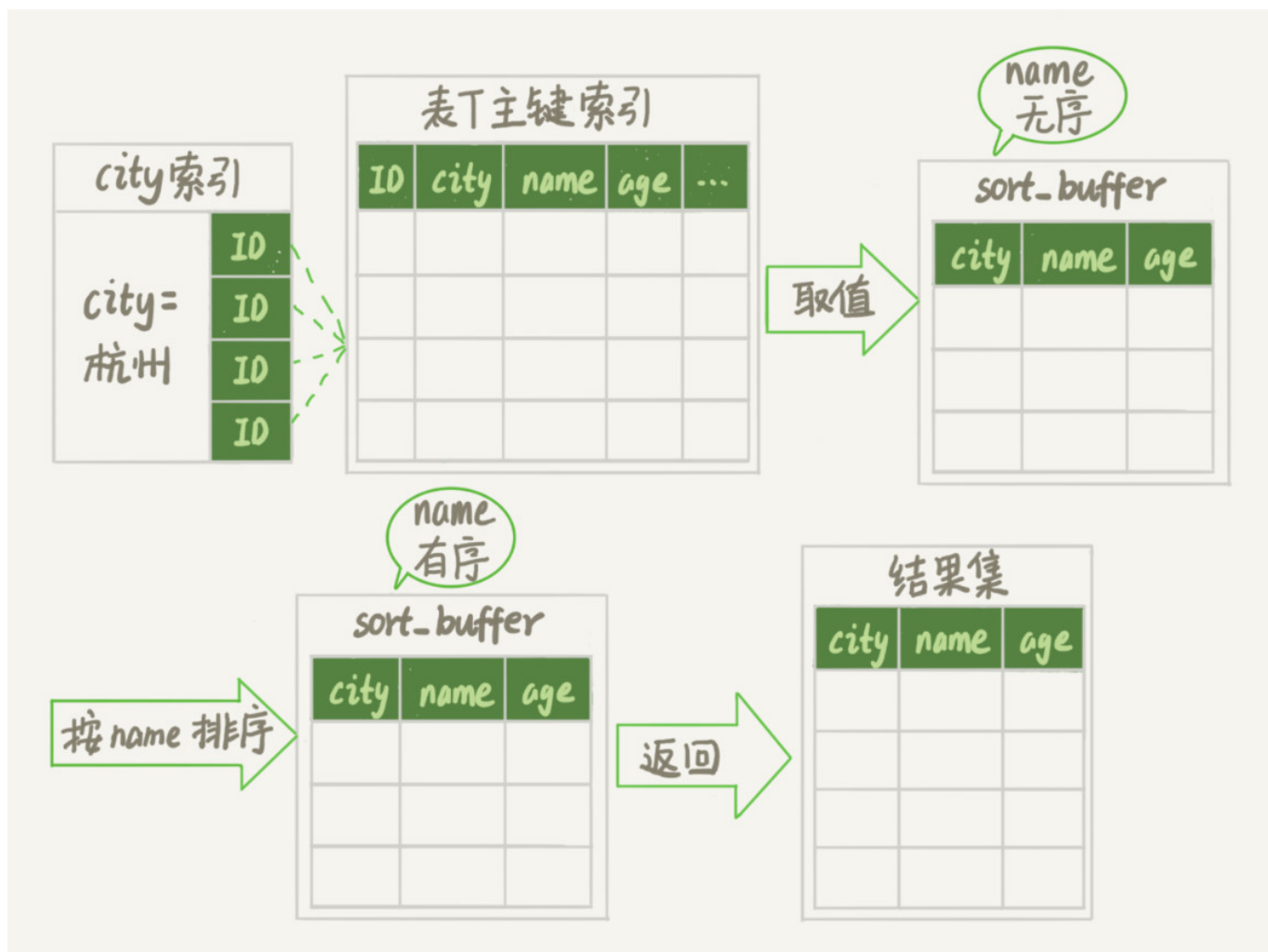
图 3 全字段排序
