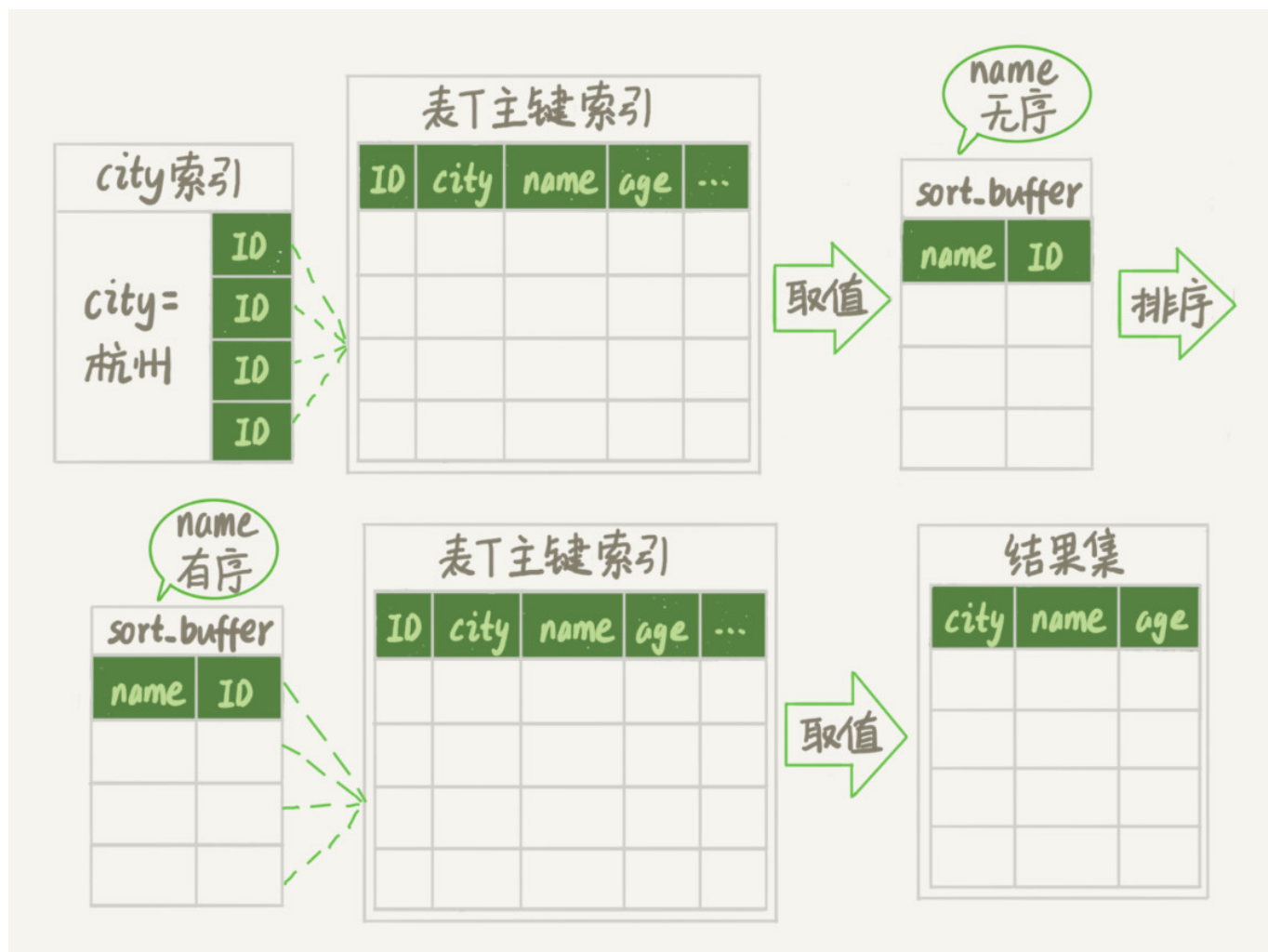
图 5 rowid 排序
